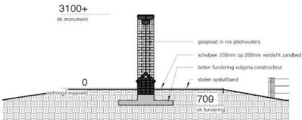
doorsnede
